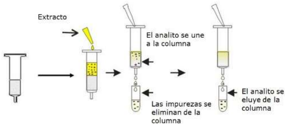
Figura 2. Procedimiento de purificación haciendo uso de columnas de inmunoafinidad (Romerlabs, 2016)
