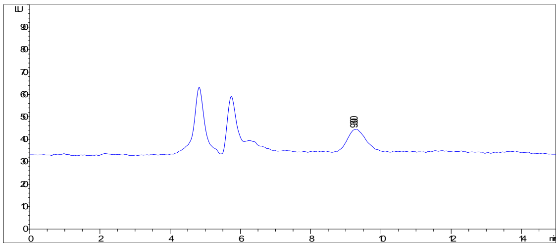
Figura 4. Cromatograma de una muestra de ración alimenticia (MPO5A) contaminada con aflatoxina G2.
