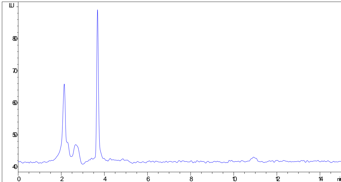
Figura 12. Cromatograma muestra blanco de leche sin enriquecer.
