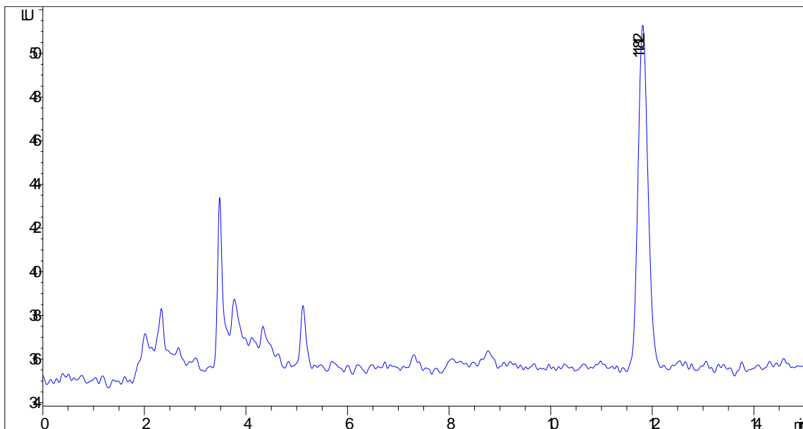
Figura 13. Cromatograma patrón M1 a 500 ng/L.
