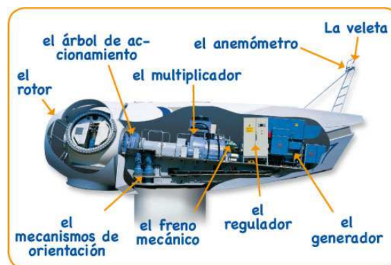
IMAGEN 1: PARTES AEROGENERADOR
