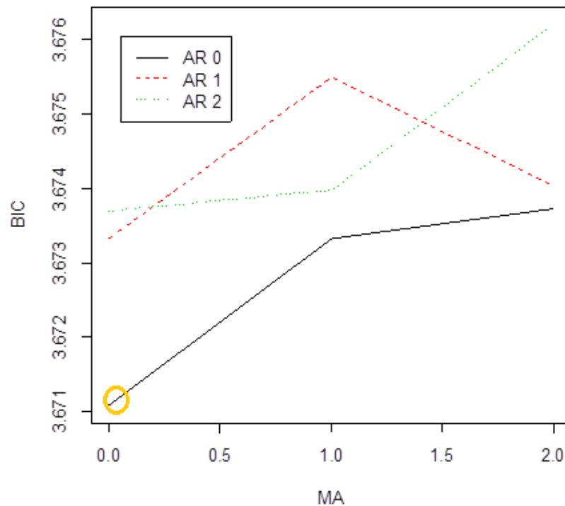
Figura 4-6: Gráfico BIC
