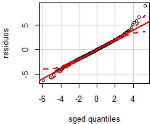
ARMA (0,0)
