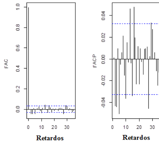
Figura 4-4: Correlograma rentabilidades
