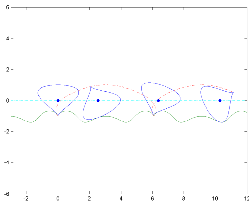
Figura 1.18: En este caso la rueda tiene forma de piriforme y su parametrización viene dada por x = \text{sen}(t) + \frac{\text{sen}(2t)}{2} , y = -\cos(t)
