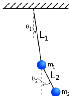
Figura 2.2: Péndulo doble
