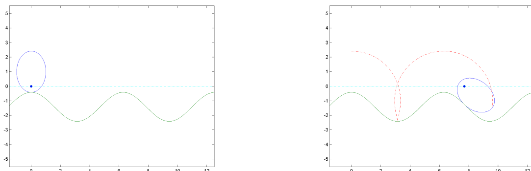
Figura 1.8: Caso k = 1 y \varepsilon = \frac{1}{\sqrt{2}} . En rojo la trayectoria del punto más alto en el momento inicial y en cyan la recta por la que se desplaza el eje
