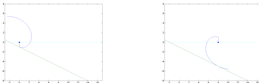
Figura 1.9: Caso n = 1, m = \frac{1}{2} . En cian la recta y = 0 por la que se desplaza el eje
