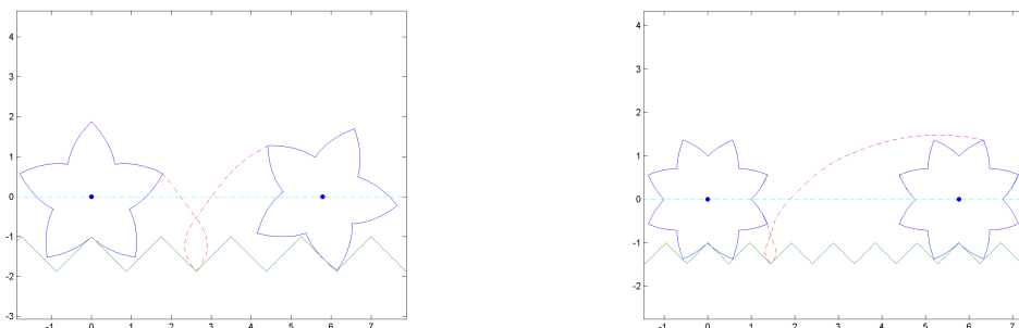
Figura 1.10: Casos n = 5 y n = 8 . En cian las rectas y = 0 por las que se desplazan los ejes
