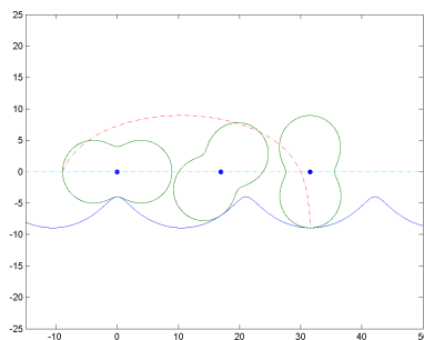
Figura 1.16: Tomando r(\theta) = 4 \sqrt{5 - 4 \sin^2(\theta)} la rueda es una curva denominada hipopede
