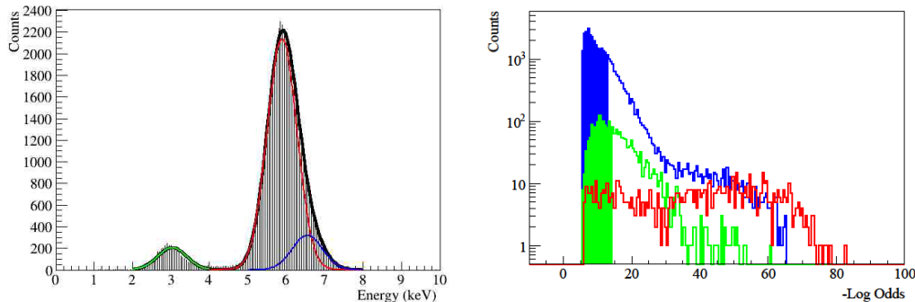
Figure 11.5: Izquierda: Espectro de ^{55}\text{Fe} en un detector Micromegas en el que se realiza el ajuste de los tres diferentes picos. Derecha: Distribución de la log-odds para el pico de 5.9 keV (azul), pico de 3 keV (verde) y eventos de fondo (rojo). El área azul corresponde al corte en 5.9 keV, mientras que el área verde corresponde al corte a 3 keV.
