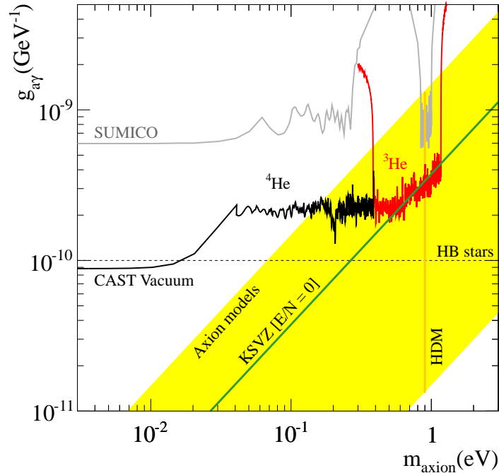
Figure 11.8: Espacio de parámetros m_a - g_{a\gamma} excluido por el experimento CAST para las fases de vacío y de {}^4\text{He} (línea negra) y los últimos resultados de la fase de {}^3\text{He} (línea roja).
