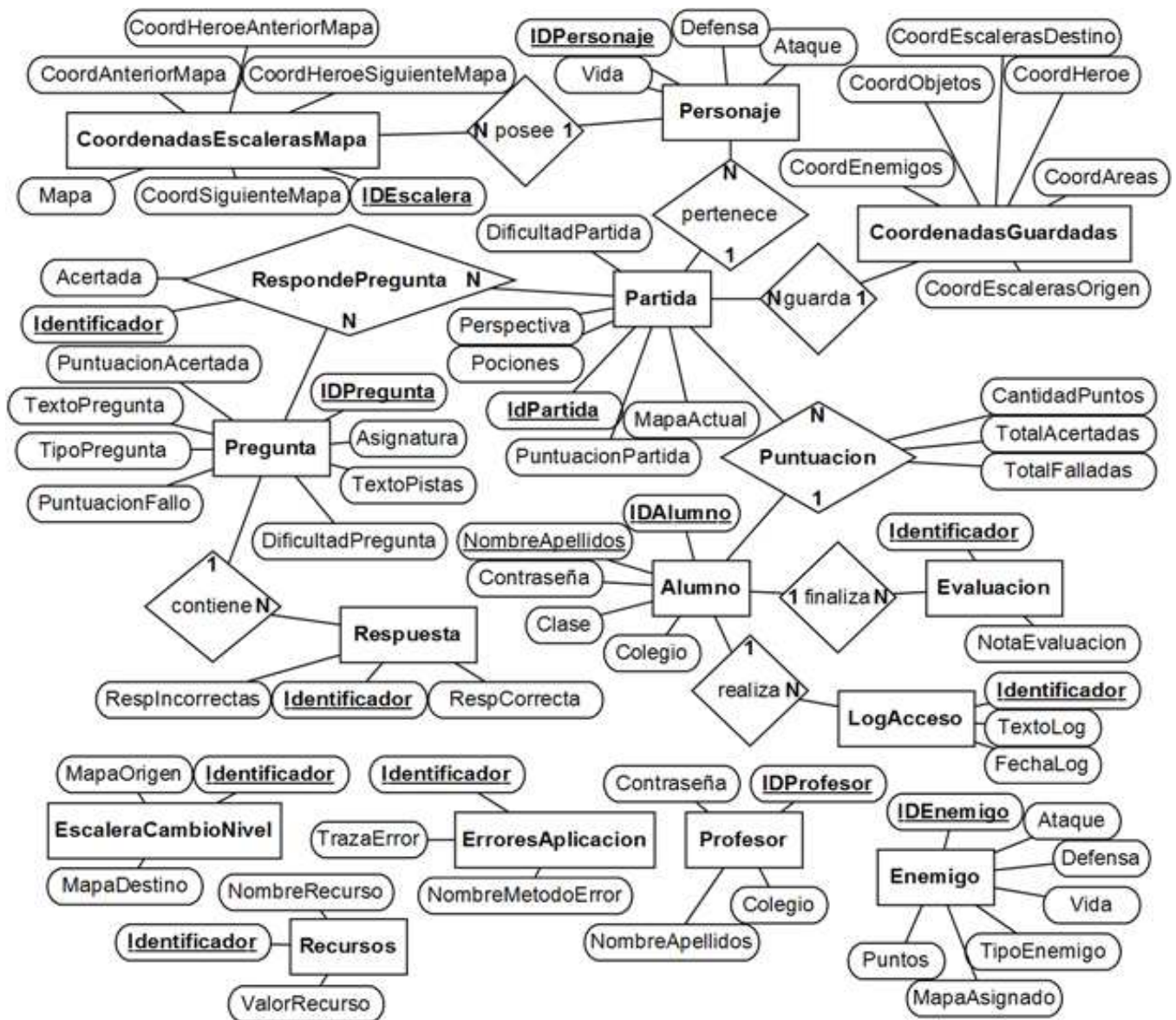
Figura 12. Diagrama entidad-relación de la base de datos.
