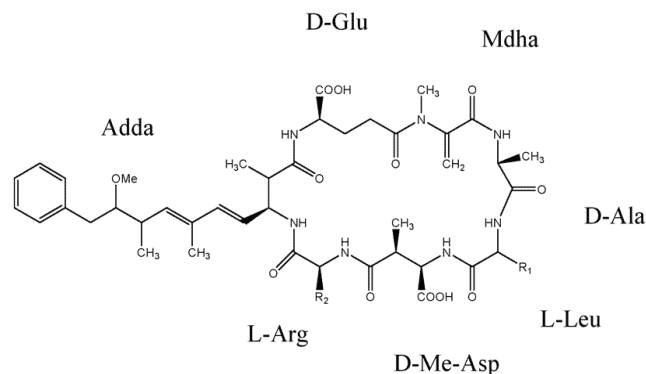
Figura 1. Variante de la cianotoxina microcistina-LR.
