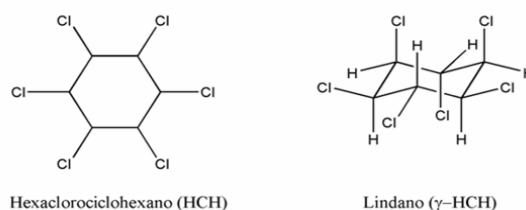
Figura 3. Fórmula química del isómero \gamma y del hexaclorociclohexano.
