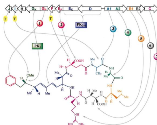
Figura 2. Estructura de operón mcy . Se puede ver la implicación de cada gen en la síntesis de la toxina.
