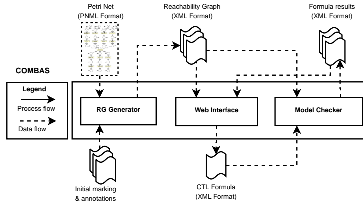
Figura 4.1: Arquitectura simplificada del framework COMBAS.
