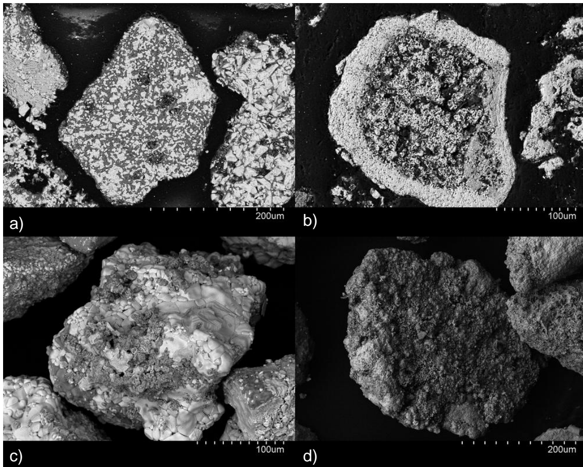
Figura 4.18: Imágenes de las partículas de TO_residuo obtenidas con microscopio SEM. Las figuras a) y b) muestran partículas cortadas y las figuras c) y d) partículas enteras; las figuras a) y c) se tomaron previamente a la combustión y las figuras b) y d) tras 88 ciclos oxidación-reducción.
