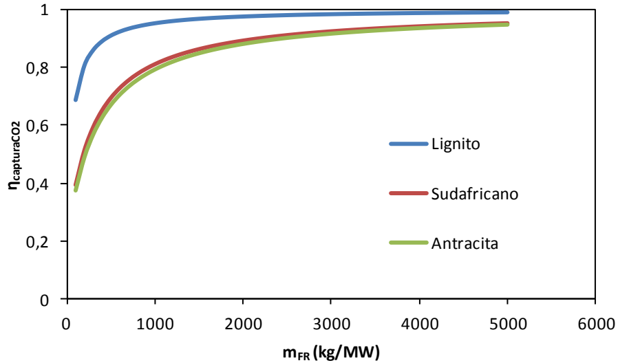
Figura 5.6: Eficacia de captura en función de m_{FR} para el TO_{residuo} alimentando los tres tipos de carbón a 900 °C, utilizando H_2O como agente gasificante.
