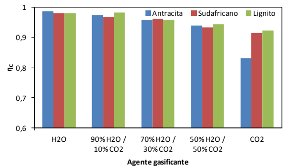
Figura 4.13: Eficacia de combustión de tres tipos de char en función del agente gasificante a 900 °C.
