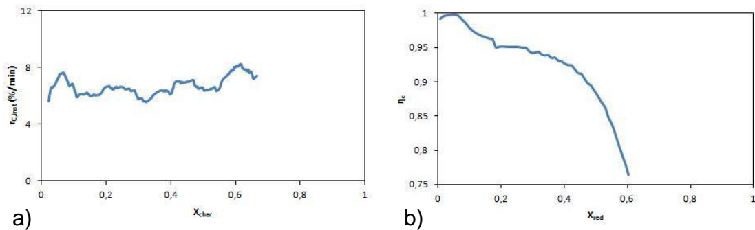
Figura 4.5: En a) se muestra la velocidad de gasificación instantánea en función de la X_{char} obtenida al realizar un experimento con char sudafricano a 900 °C utilizando H 2 O como agente gasificante con un lecho de 2,5% de TO_mineral en alúmina y en b) la eficacia de combustión frente a X_{red} obtenida en el mismo experimento.
