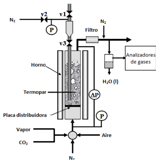
Figura 3.1: Esquema de la instalación empleada.
