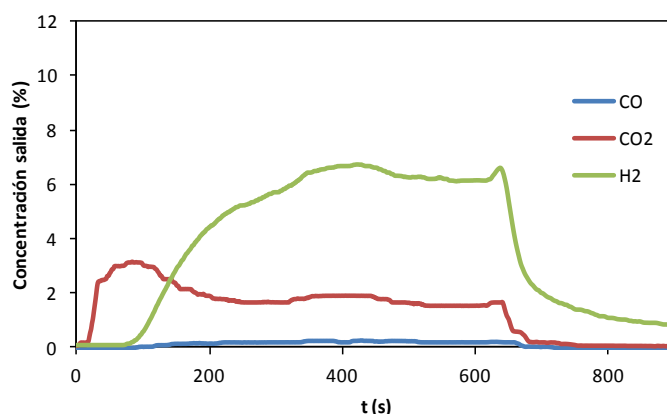
Figura 4.20: Composición de la corriente de salida con respecto al tiempo de un experimento con char de carbón sudafricano a 900 °C utilizando H 2 O como agente gasificante con un lecho de 5% de TO_sintético.
