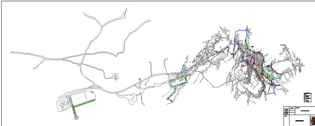
Figura 4: Red de Pluviales de Albalate del Arzobispo
