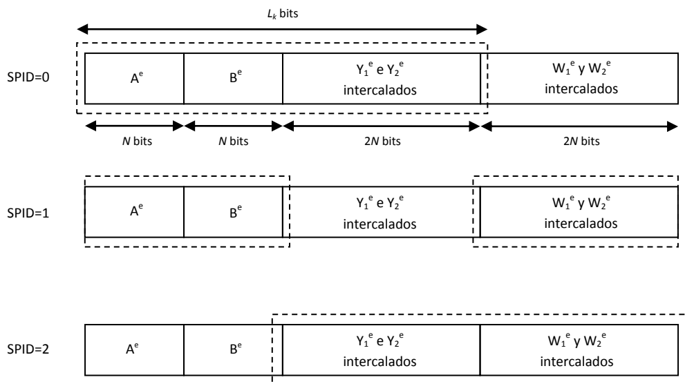
Figura 13. Proceso de puncturing para HARQ tipo II - IR con 2 retransmisiones y tasa de código global 1/2
