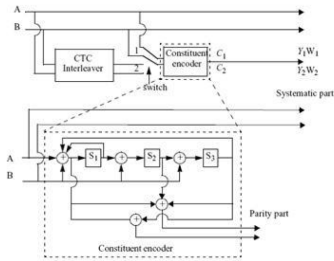
Figura 10. Codificador CTC
