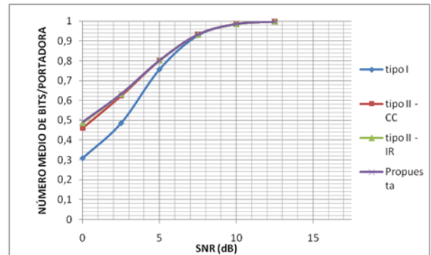
Figura 23.b. Eficiencia para QPSK, tasa 1/2, bloque de 36 bytes y canal Vehicular A
