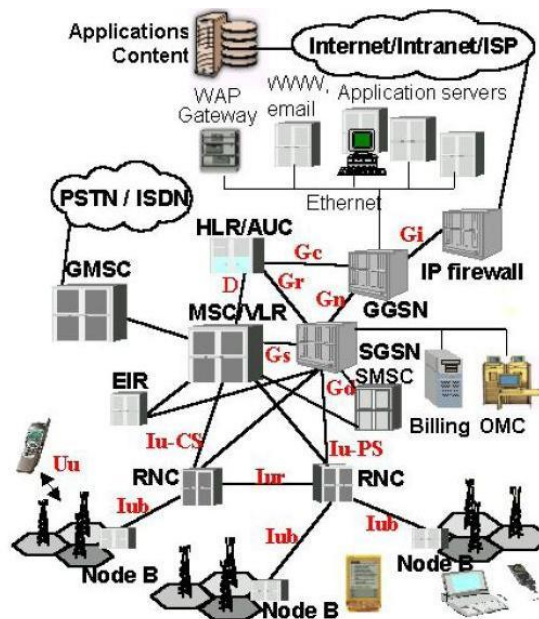
Figura 3. Arquitectura del sistema UMTS
