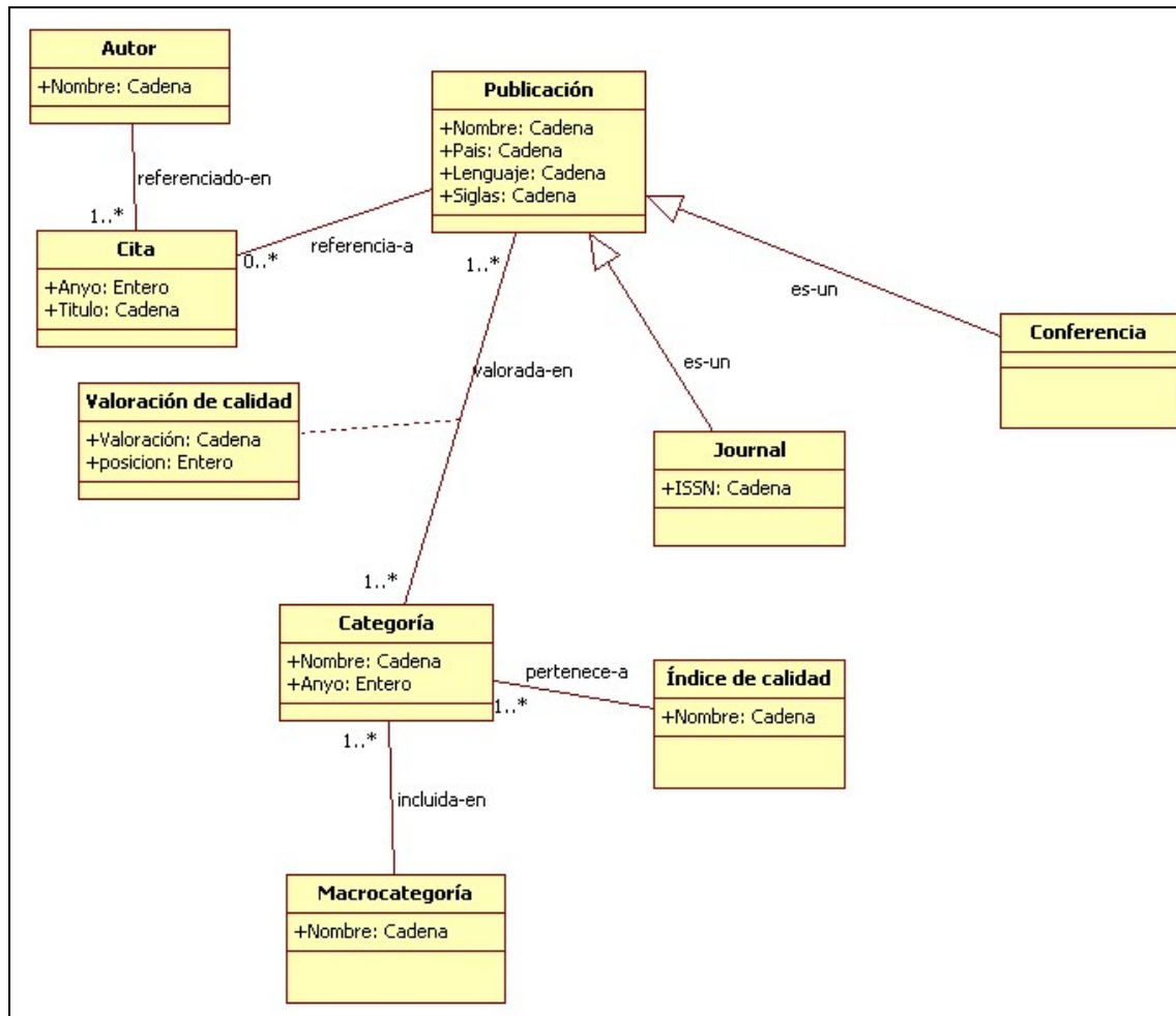
Figura 5: Modelo de dominio del análisis
