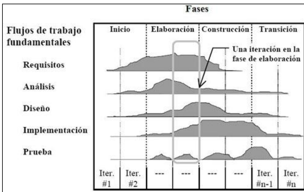
Figura 1: Fases del Proceso Unificado
