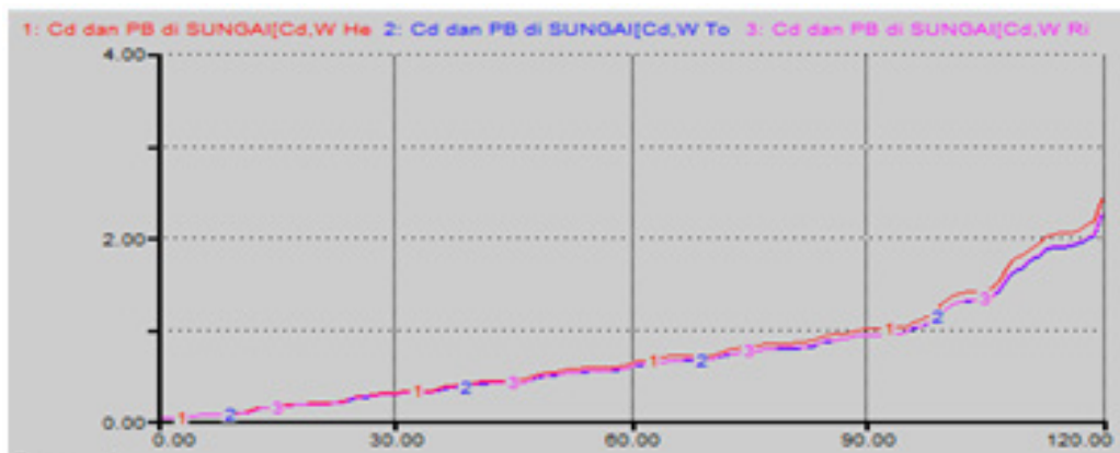
Gambar 4. Estimasi Konsentrasi Cd (2015 – 2025) Berdasarkan Skenario 3 di 3 Sungai
