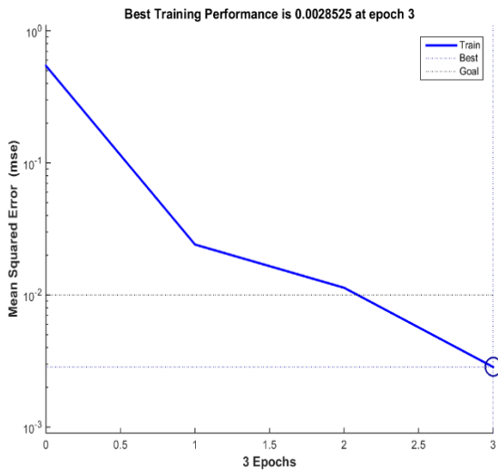
Gambar 7. Error MSE pada JST dengan 13 Hidden Node
