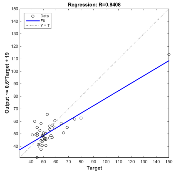
Gambar 8. Hasil Uji Regresi JST dengan 13 Hidden Node
