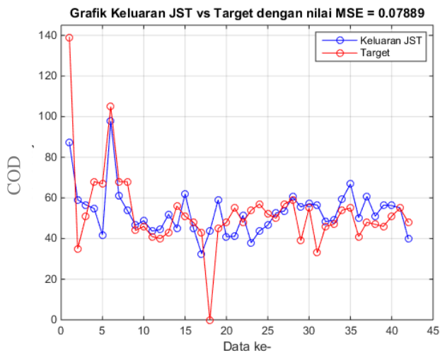
Gambar 7. Hasil validasi Model JST
