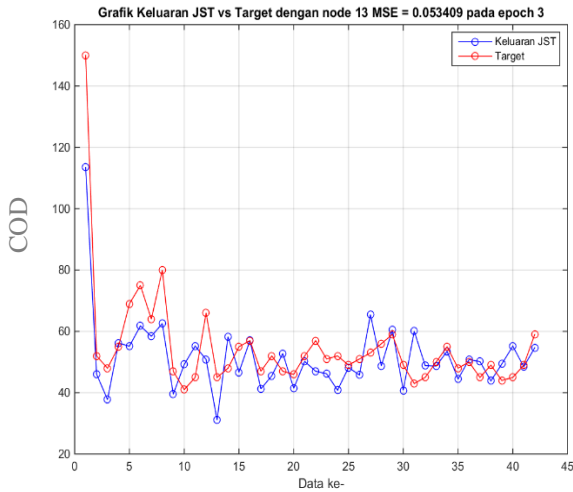
Gambar 6. Hasil training keluaran JST terhadap Target
