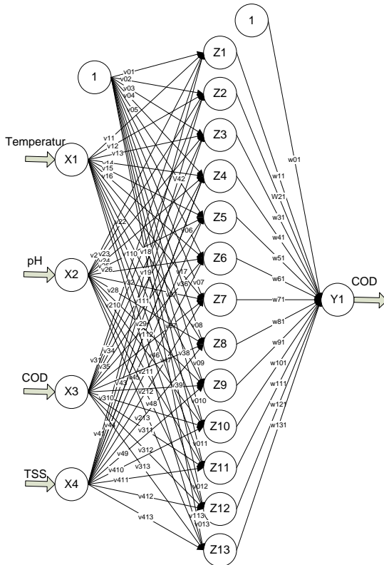
Gambar 3. Arsitektur JST pada keluaran COD
