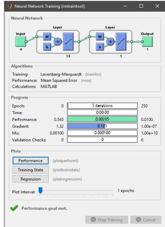
Gambar 5. nntaintool hidden node 13
