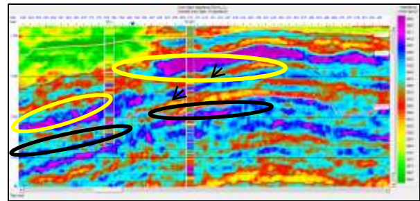
Gambar 4 Hasil Inversi Impedansi
