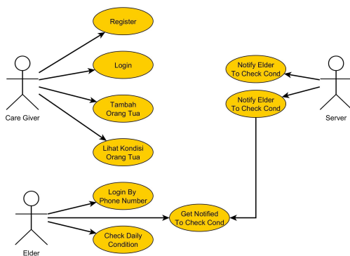
Gambar 3. Aktifitas yang dapat dilakukan setiap entitas sesuai dengan dukungan sistem.
