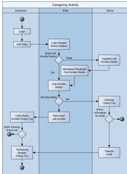
Gambar 5. Diagram aktivitas caregiving antara caregiver, elder, dan server.
