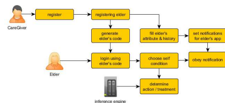
Gambar 2. Alur Tindakan pemanfaatan sistem yang dapat dilakukan oleh pengguna
