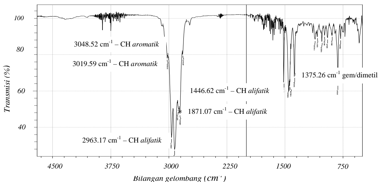
Gambar 2. Spektrum inframerah isolat CXA
