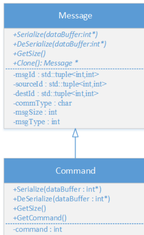
Fig. 23. Command Message Class Diagram.
