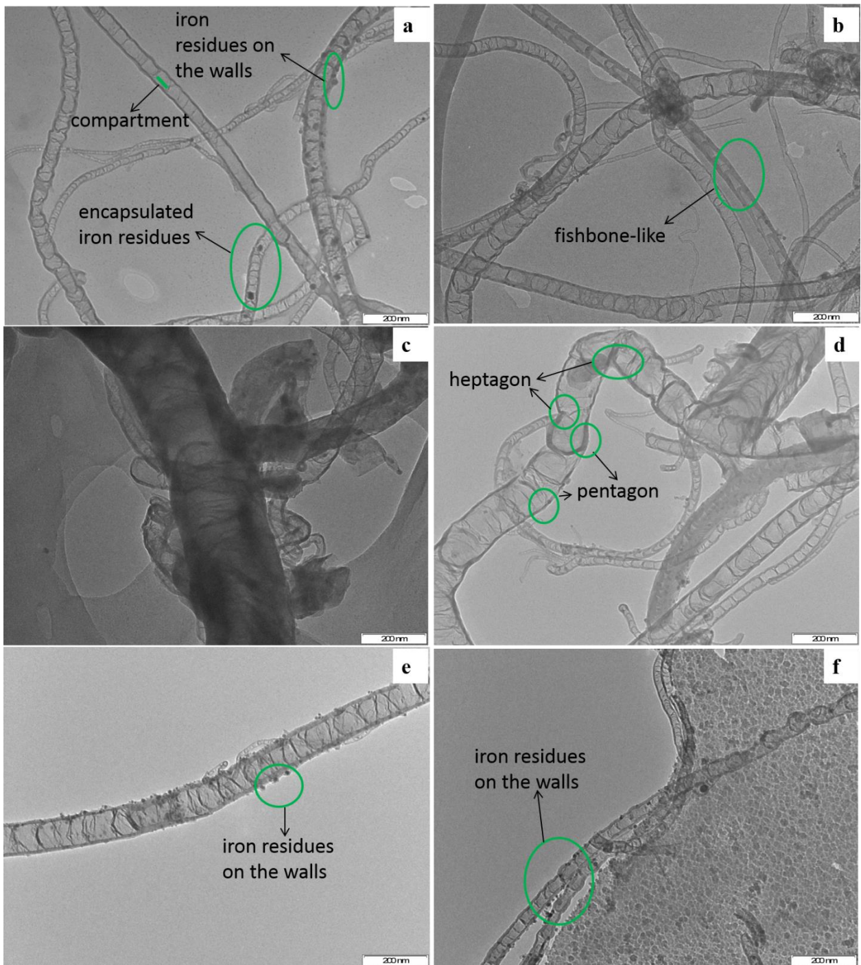
Fig. 3.2. Representative TEM images for the D1Ax samples (a) D1A0, (b) D1A1, (c) D1A2, (d) D1A3, (e) D1A4 and (f) D1A5.
