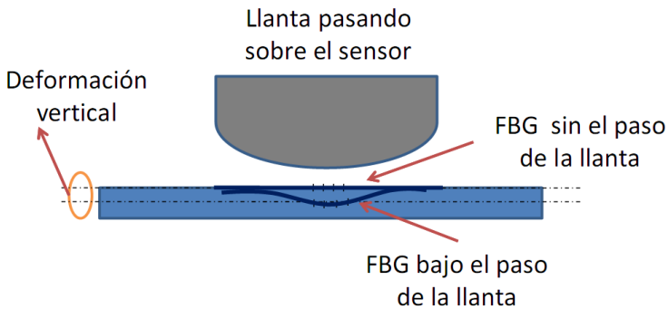
Figura 5: representación gráfica del paso de la llanta sobre el sensor FBG. La figura inserta muestra una ampliación en 6000x de la deformación en la superficie según la simulación con el MEF
