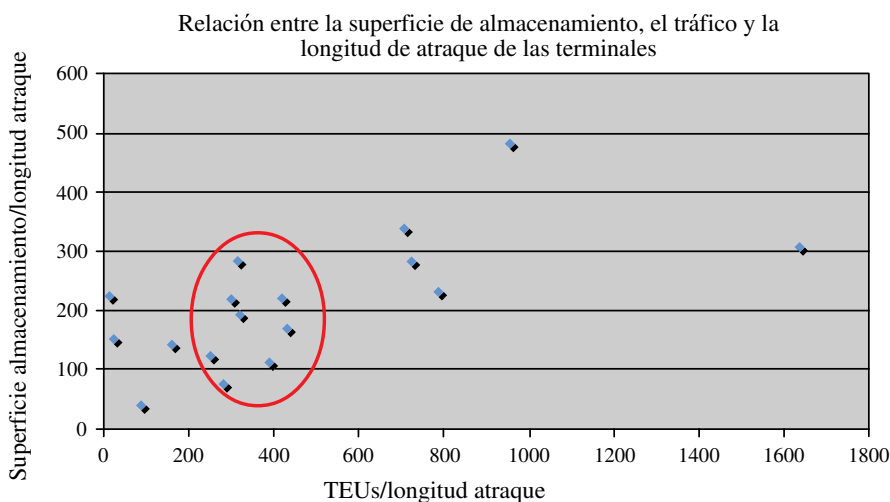
Figura 15: relación entre la superficie de almacenamiento, el tráfico y la longitud de atraque de terminales de contenedores del sur de Europa
