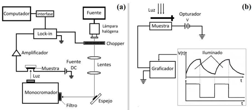
Figura 3: (a) Diseño experimental para las medidas de fotoconducividad. (b) Circuito empleado para medir la variación del foto-voltaje en el tiempo y determinar el tiempo de respuesta de las películas delgadas de ZnSe.
