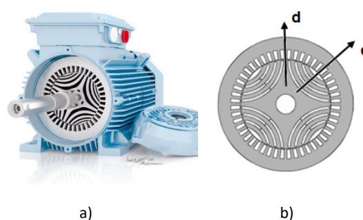
Figura 6 – MSrel: a) aspeto geral; b) corte seccional
