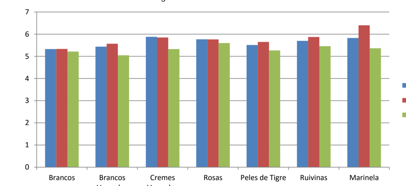
Figura 6 - Provetes saturados.
