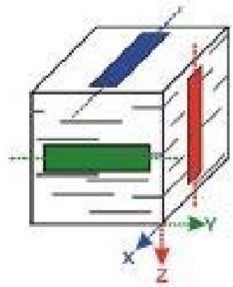
Figura 2 - Planos de medição segundo os três eixos ortogonais.
