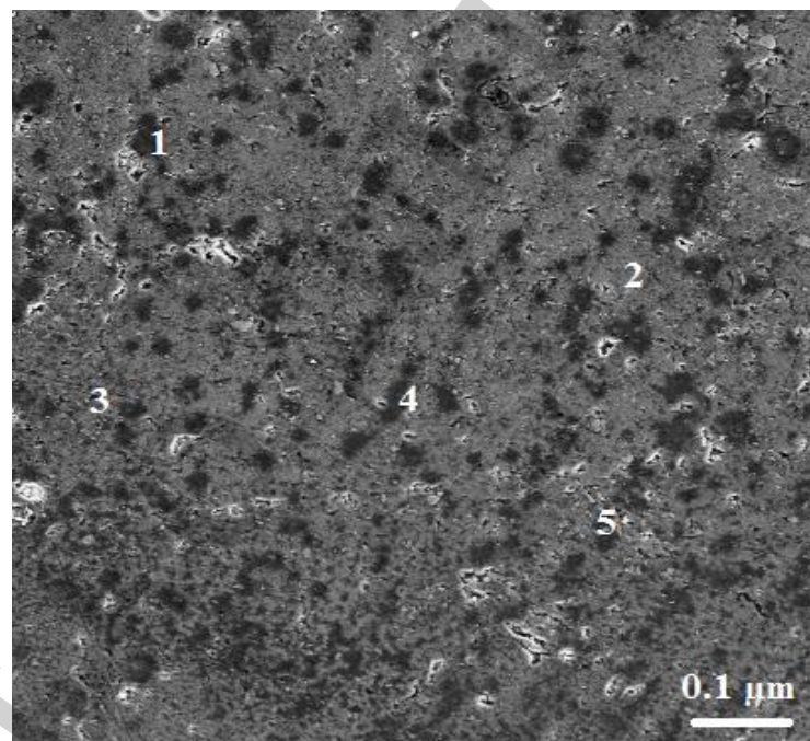
Рис. 1. Структура композиту AM4,5Кд+10 % MoS 2 : a – представлено розподіл MoS 2 , вказано стрілками, шліф не травлений; б – зображення інтерметалідів (1 – CuAl 2 , 2 – MnAl 6 , 3 – NiAl 3 , 4 – TiAl 3 , 5 – Al 2 CuMn), шліф травлений (NaOH). Зображення отримано на металографічному мікроскопі
