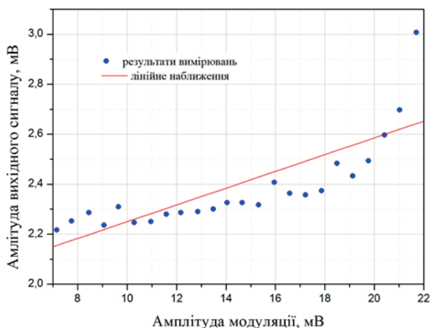
Рис. 5. Зміна амплітуди вихідного сигналу при зміні амплітуди модуляції в діапазоні 0–15 мВ. Частота сигналу модуляції становила 30 Гц
