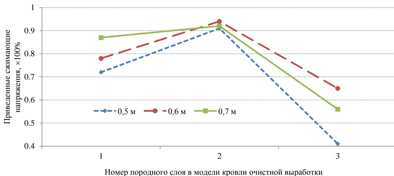
Рис. 3. Изменение приведенных максимальных сжимающих горизонтальных напряжений по породным слоям на плоскости очистного забоя в средней части очистной выработки при сплошной закладке с различной высотой пресекаемых пород
