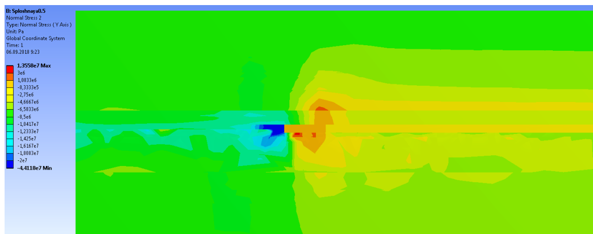
Рис. 2. Вертикальные напряжения в поперечном разрезе на расстоянии 0,5 м от выемочной выработки при сплошной закладке с высотой пресекаемых пород 0,5 м
