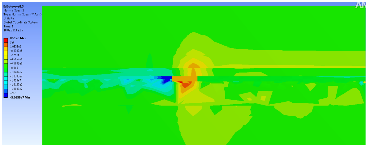
Рис. 1. Вертикальные напряжения в поперечном разрезе на расстоянии 0,5 м от выемочной выработки при закладке бутовыми полосами с высотой пресекаемых пород 0,5 м.
