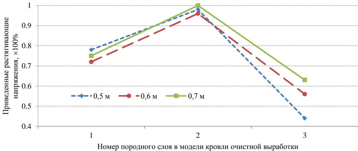
Рис. 4. Изменение приведенных максимальных растягивающих горизонтальных напряжений по вертикали на плоскости очистного забоя в средней части очистной выработки при сплошной закладке с различной высотой пресекаемых пород
