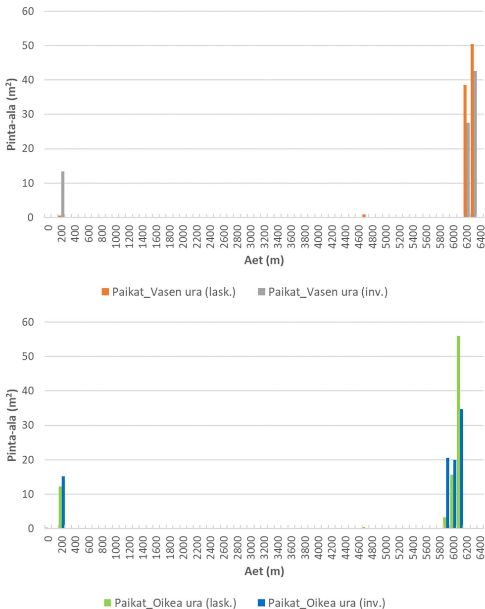
Kuva 5. Kohteen A yhden tieosan kuvista inventoitujen ja karkeusdatasta laskettujen valuasfalttipaikkojen vertailu vasemmalle ja oikealle ajouralle.
