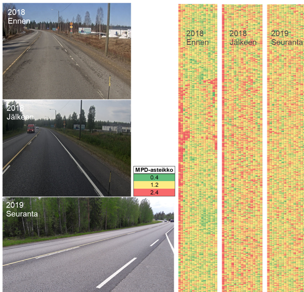
Kuva 19. Kohteen C yhdeltä tieosalta ennen päällystystä havaitun karkean kohdan seuranta. Vuoden 2019 valokuva on otettu maastokäynnin yhteydessä. Kuvan oikean reunan 10 cm MPD-tulokset ovat 40 m matkalta (Aet 1840-1880 m).
