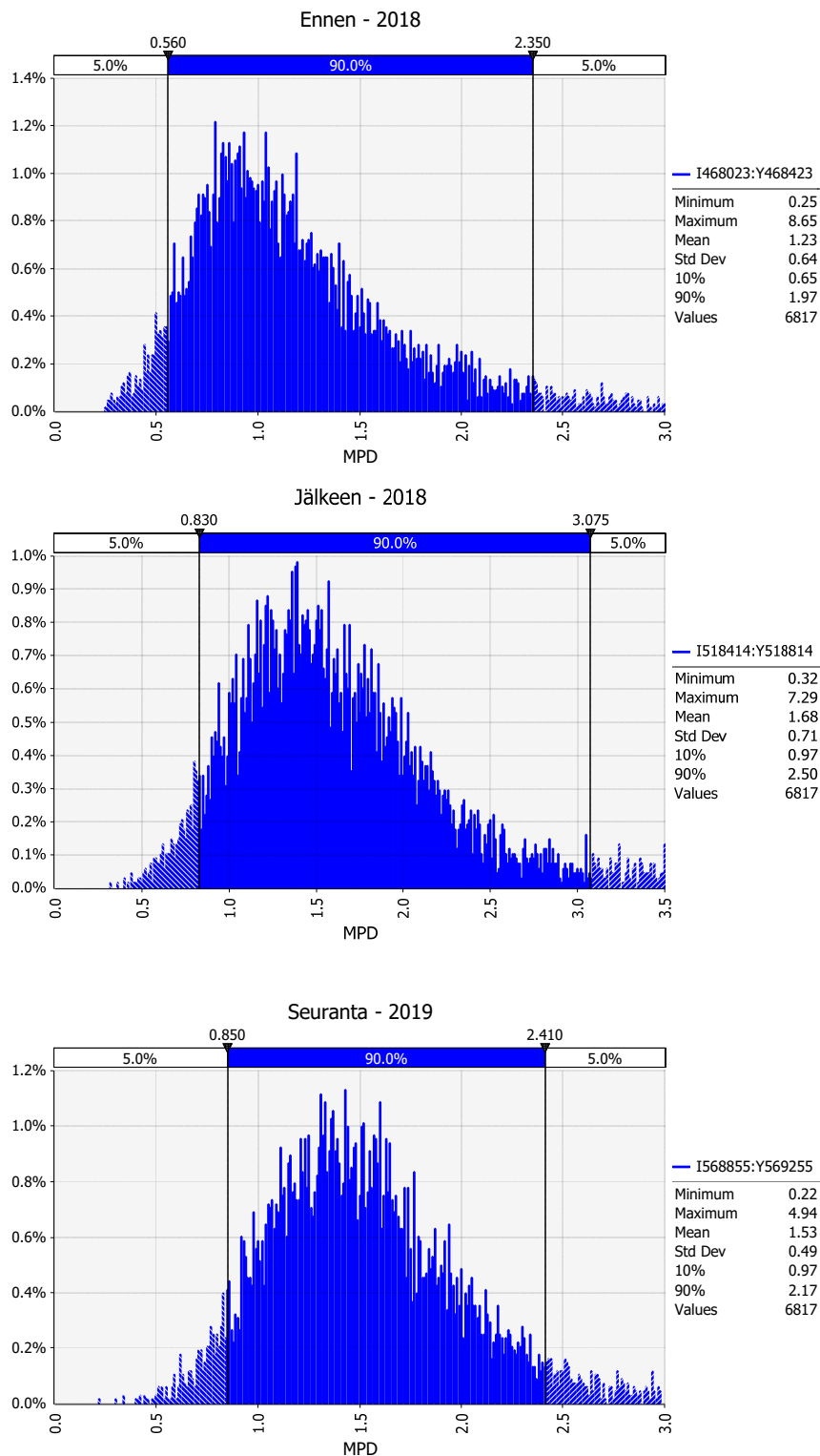
Kuva 23. Pinnan karkeuden muutos 10 cm MPD-tulosten histogrammiin ja muutamien tilastollisten tunnuslukujen avulla ennen toimenpidettä (yllä), toimenpiteen jälkeen (keskellä) ja ensimmäisen talven jälkeen (alla) kuvan 22 kohtaa vastaavalta matkalta (Aet 4560–4600 m). Huomaa keskimäisen kuvan MPD-asteikko verrattuna muihin kuviin.
