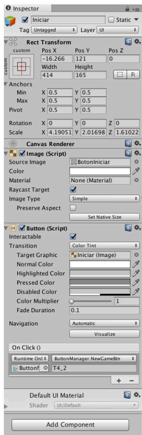
Ilustración 53: Inspector del botón Iniciar
