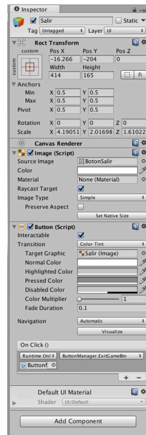
Ilustración 54: Inspector del botón Salir
