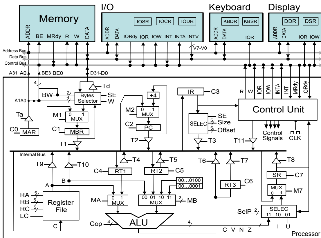
Figura 2-7: Arquitectura CPU WepSIM.
