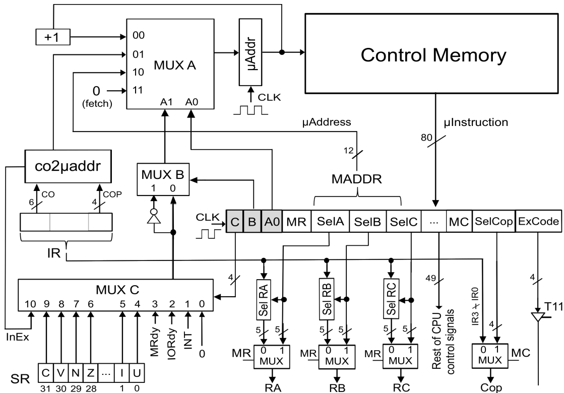
Figura 2-8: Arquitectura unidad de control WepSIM.
