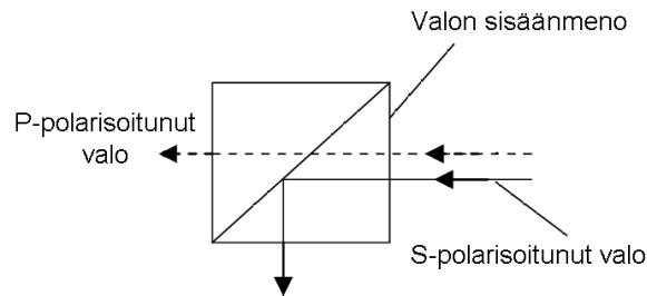
Kuva 10. Polaarisuuden perusteella toimiva säteenjakaja, PBS [1, s. 377].
