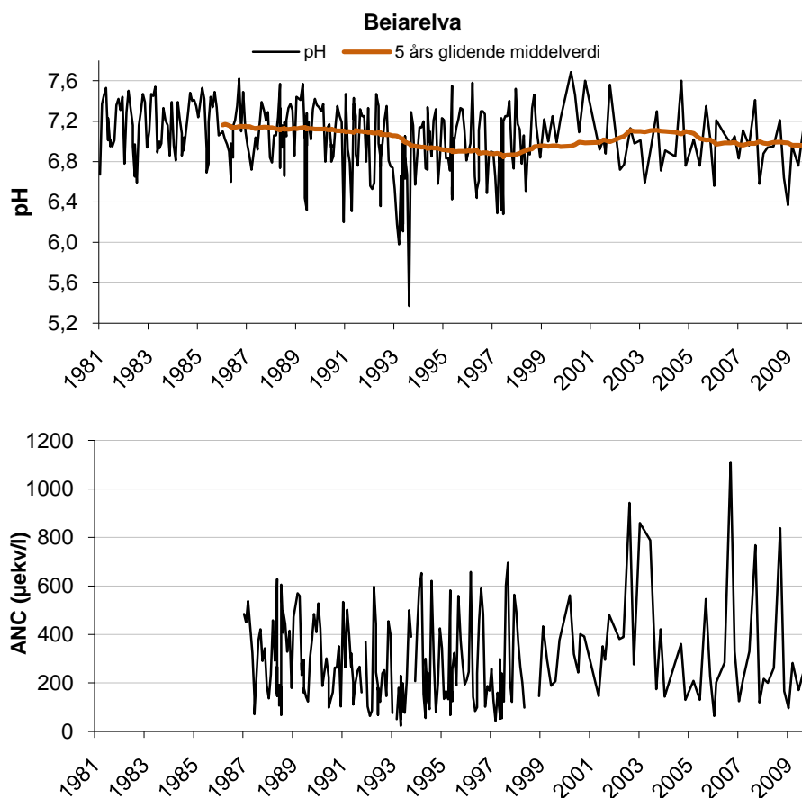
Figur 10. pH med 5 års glidende middelværdi og ANC i Beiarelva i perioden 1981-2009.
