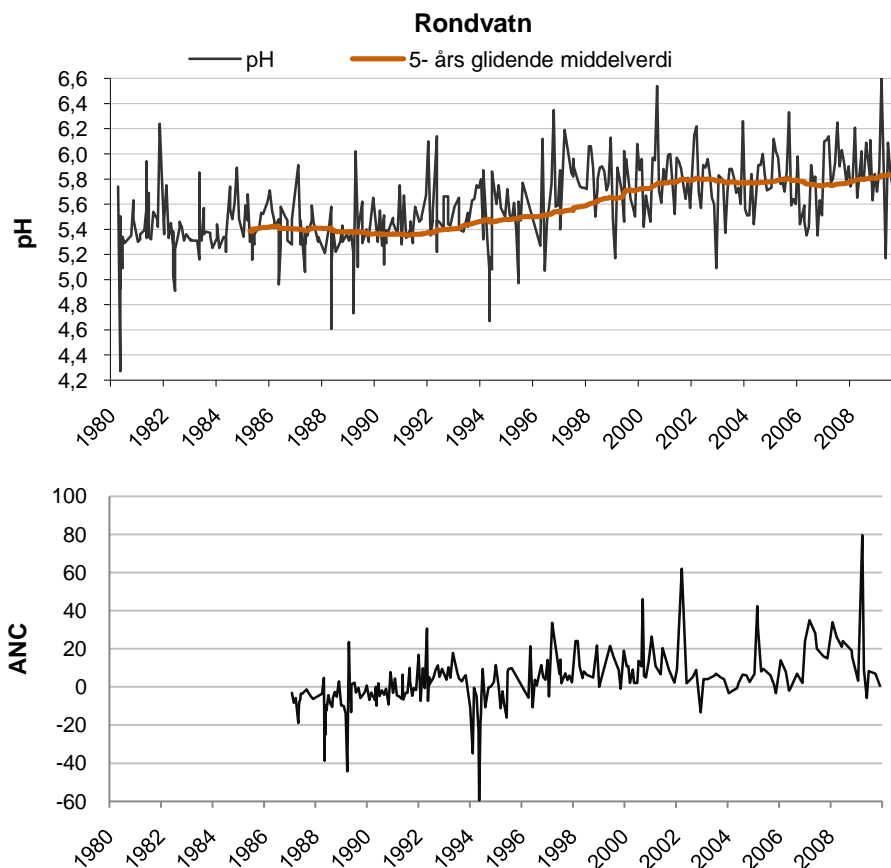
Figur 2. pH med 5 års glidende middelværdi og ANC i Rondvatn i perioden 1980-2009.
