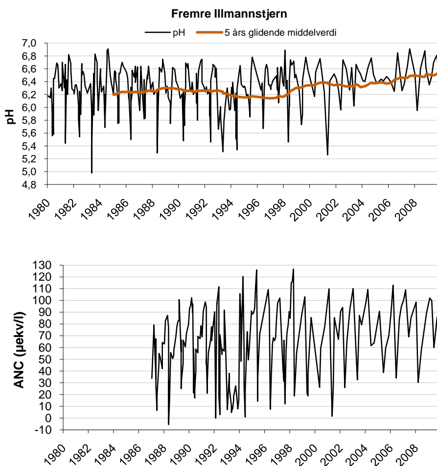
Figur 4. pH med 5 års glidende middelværdi og ANC i Fremre Illmanntjern i perioden 1980-2009.
