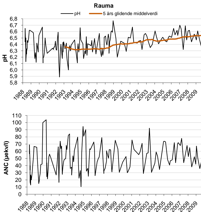
Figur 17. pH med 5 års glidende middelvei og ANC i Rauma i perioden 1988-2009.
