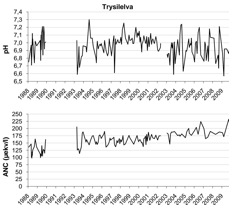
Figur 14. pH og ANC i Trysilelva i perioden 1988-2009.
