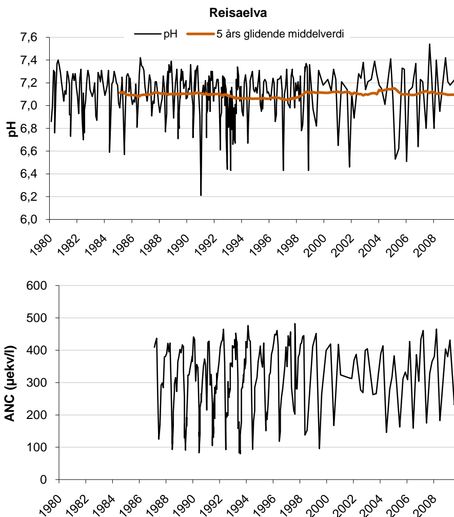
Figur 11. pH med 5 års glidende middelværdi og ANC i Reisaelva i perioden 1980-2009.
