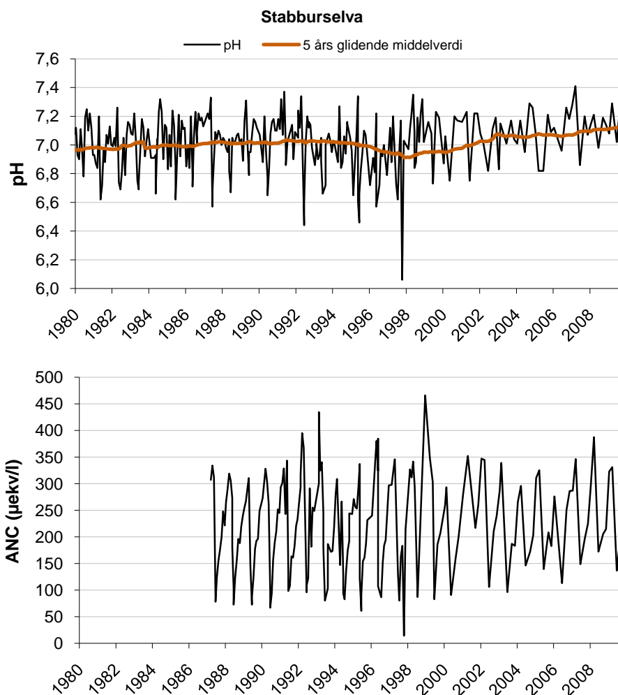
Figur 13. pH med 5 års glidende middelværdi (dataserien starter i 1973) og ANC i Stabburselva i perioden 1980-2009.
