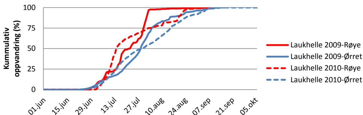
Figur 43. Kumulativ oppvandring av sjørøye og sjørret i Laukhellevassdraget i 2009 og 2010.
