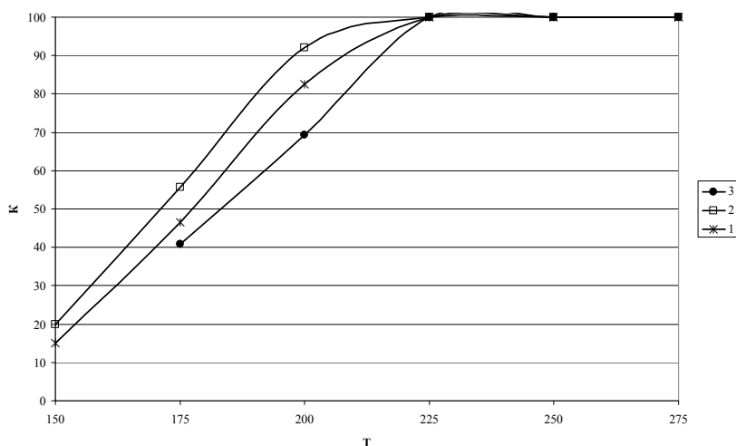
Рис. 1. Зависимость конверсии водно-метанольной смеси от температуры.
