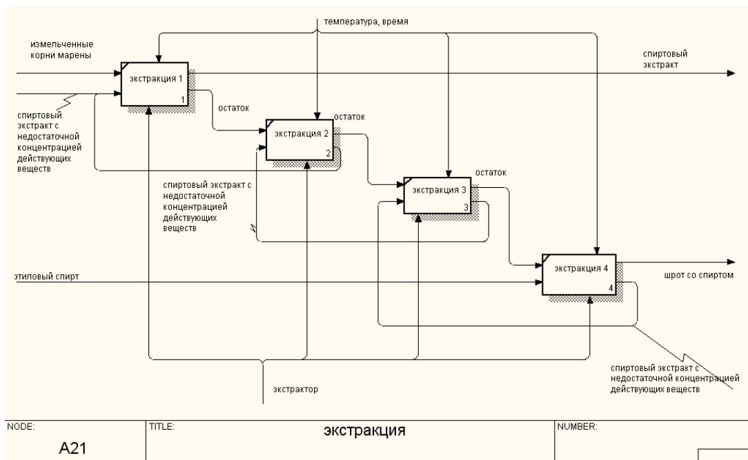
Рис. 4. Функциональная диаграмма, описывающая процесс псевдонепрерывной противоточной экстракции.
