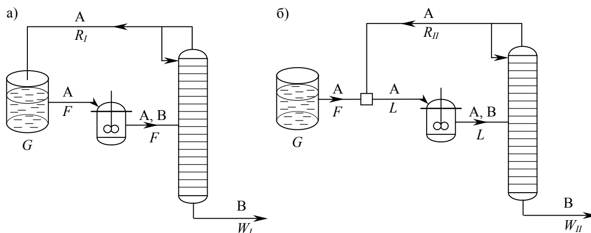
Рис. 1. Способы организации рецикла по реагенту А.
