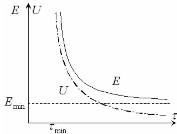
Рис. 2. Зависимость парового потока и суммарных затрат от времени проведения процесса.
