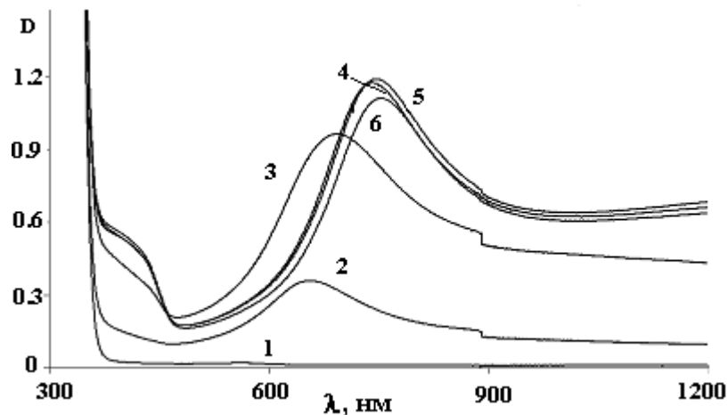
Рис. 1. Электронные спектры поглощения растворов при полимеризации анилина. [H^+]/[Анилин] = 8.21 г-экв/моль. Время полимеризации: 0 (1), 20 (2), 25 (3), 30 (4), 35 (5) и 50 мин. (6).
