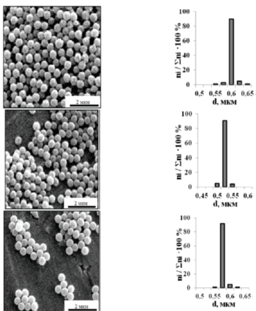
Рис. 11. Микрофотографии и гистограммы распределения по размерам частиц полистирольных суспензий, полученных при различных концентрациях ПДМС-эпокси-30: 1 – 0.1% мас. 2 – 2.0% мас.; 3 – 5.0%
