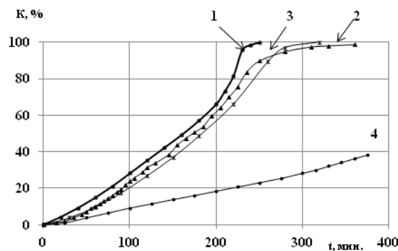
Рис. 3. Кривые конверсия – время, полученные при полимеризации стирола в присутствии 1% мас. ПАВ: 1 – ПДМС-эпокси-30; 2 – ПДМС-NH 2 -30; 3 – ПДМС-СООН-30; 4 – полимеризация в массе.
