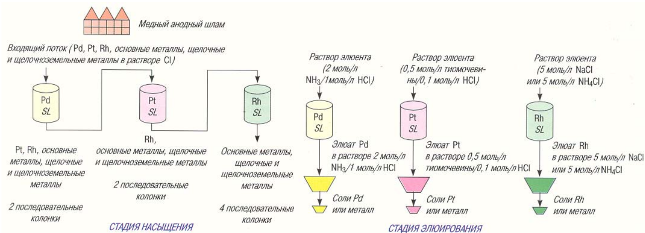
Рис. 6. Технологическая схема получения палладия, платины и родия методом ТМР.
