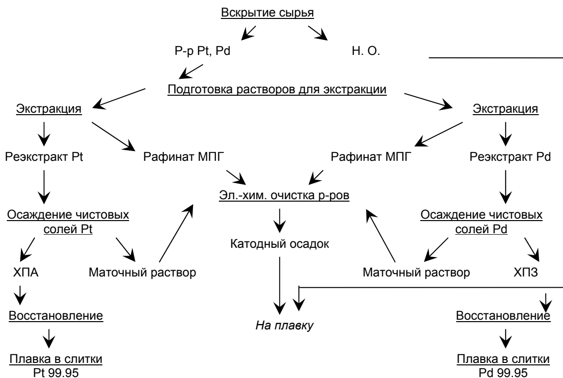
Рис. 4. Технологическая схема получения слитков платины и палладия с использованием экстракционных переделов (здесь МПГ – металлы платиновой группы; Н.О. – нерастворимый остаток; ХПА – (\text{NH}_4)_2[\text{PtCl}_6] ; ХПЗ – транс - [\text{Pd}(\text{NH}_3)_2\text{Cl}_2] ).
