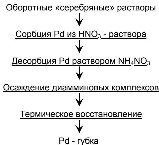
Рис. 5. Идея получения палладия аффинированного с использованием сорбционного передела.
