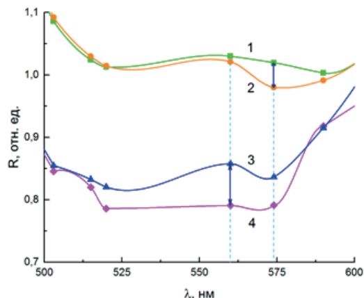
Рис. 3. Спектры диффузного отражения адсорбированных на ММК реагента пикрамина-ε и его комплексов с Cu(II): 1 – C_{п-ε} = 0.04 мкг/см 3 ; 2 – C_{Cu(II)} = 0.01 мкг/см 3 ; 3 – C_{п-ε} = 0.4 мкг/см 3 ; 4 – C_{Cu(II)} = 0.1 мкг/см 3 . V = 50 см 3 , скорость пропускания 20 см 3 /мин, рН 1.
