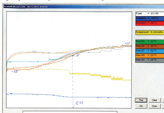
Рис 2. График лиофилизации (зависимость температуры препарата от времени) липосомального гентамицина по предложенной программе.
