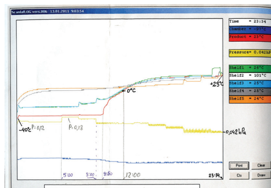
Рис. 1. График производственной сушки (зависимость температуры препарата от времени), сопровождавшейся резким подъемом температуры препарата.
