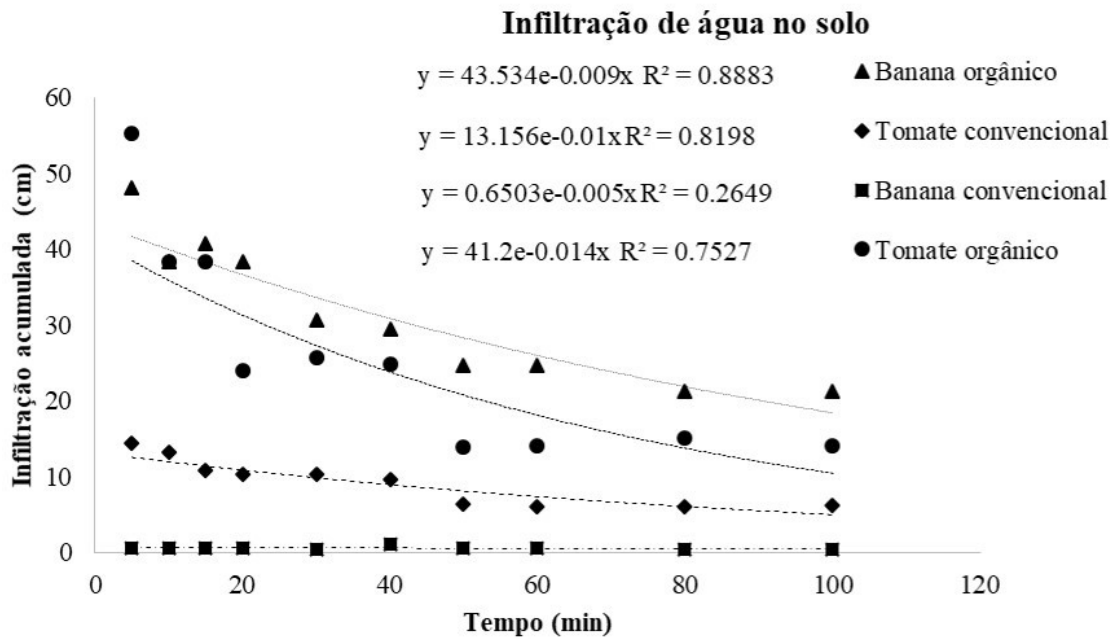
Figura 1: Velocidade de infiltração de água no solo em função de diferentes usos e manejo do solo.
