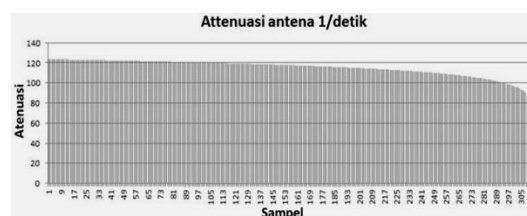
Gambar 5 Grafik Atenuasi Antena 1 Per Detik
