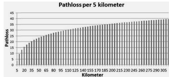
Gambar 6 Grafik Pathloss Per 5 Kilometer
