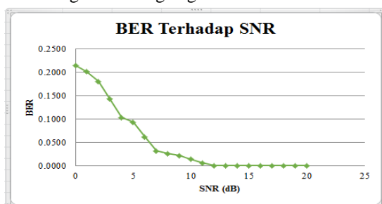
Gambar 3. Grafik SNR Terhadap BER Pada MIMO-OFDM
