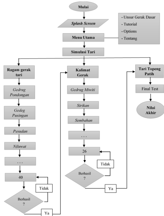
Gambar 10. Alur Program Aplikasi
