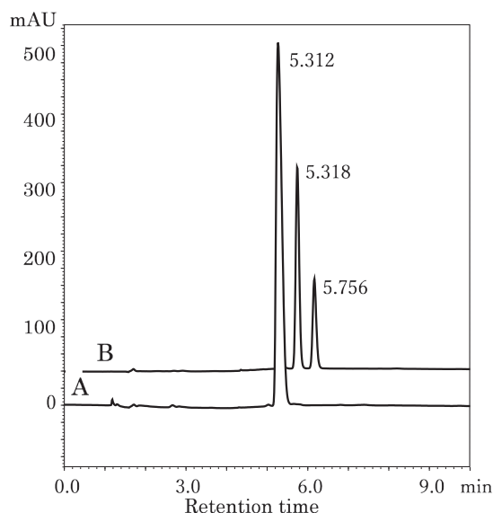
図2 スリンダクのHPLCクロマトグラム (A) 紫外線照射前 (B) 紫外線照射後
