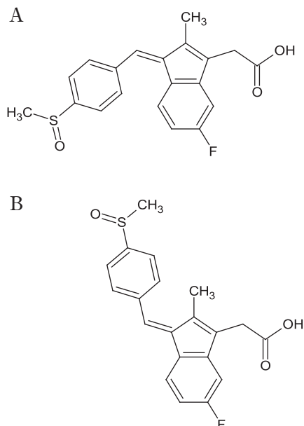
図1 スリダク (A) とその光分解物 (B) の化学構造
