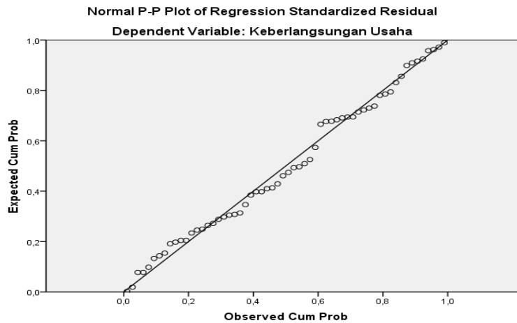
Gambar 1. Pengujian Normalitas Menggunakan Grafik P-P Plot Sumber: Hasil Penelitian 2018
