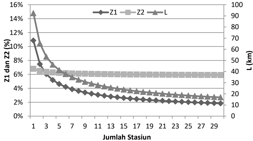
Gambar 5. Grafik Z1, Z2 dan L
