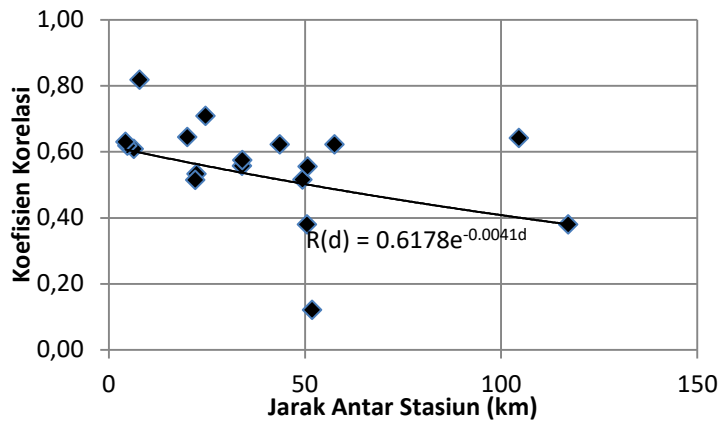
Gambar 4. Grafik Hubungan Jarak Setiap Stasiun dan Koefisien Korelasi dari Jarak Stasiun
