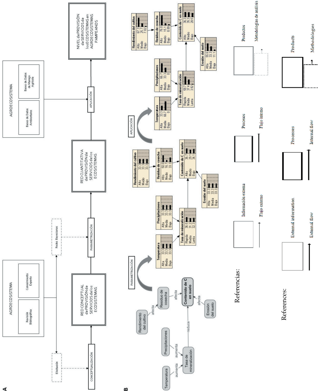
Figura 1. A) Representación esquemática del proceso lógico de desarrollo del nuevo marco analítico de evaluación de la provisión de servicios de los ecosistemas en los agroecosistemas pampeanos basado en redes conceptuales y redes probabilísticas. En el esquema se representan los pasos principales junto con la metodología de análisis y la información externa necesaria para obtener los productos principales de cada etapa. B) Ejemplo de los productos principales de cada etapa del nuevo marco analítico en base al servicio del ecosistema balance de C del suelo. En la etapa de parametrización sólo se presenta el resultado de la elicitación del conocimiento experto en aquellas variables dependientes de una o más variables. La etapa de aplicación se ejemplifica con información ambiental y productiva correspondiente a la zona sur de Entre Ríos para el cultivo de maíz durante la campaña 2000/2001.
