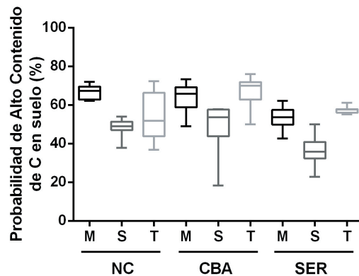
Figura 2. Respuesta probabilística de la variable respuesta alto contenido de C en suelo, correspondiente al servicio del ecosistema balance de C del suelo, en relación a las tres zonas agrícolas bajo estudio. En cada caja se representan los cuartiles Q1 (25% de los datos), Q2 ó mediana (50% de los datos) y Q3 (75% de los datos). Los bigotes representan los valores mínimo y máximo de cada situación. Referencias: M=maíz, S=soja, T=trigo, NC=norte de Córdoba, CBA=centro de Buenos Aires, SER=sur de Entre Ríos.
