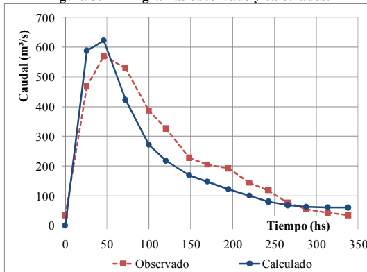
Figura 6: Hidrogramas observado y calculado.
