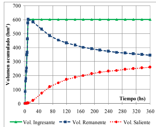
Figura 7: Variación temporal de volúmenes acumulados.
